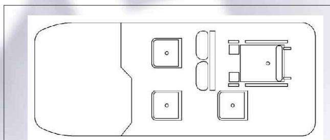
Schema abitabilità con 1 carrozzina.
